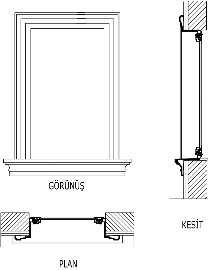
- PREKAST MONTAJ DETAYI -
